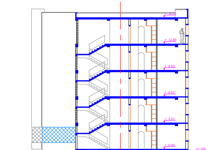
Coupe AA
